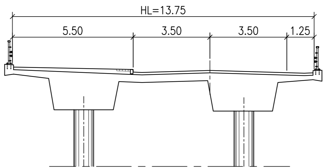
POIKKILEIKKAUS 1:100
