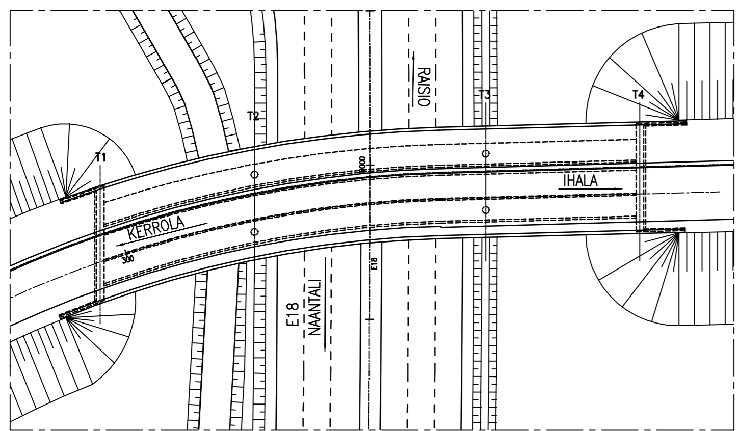
TASOKUVA 1:500
